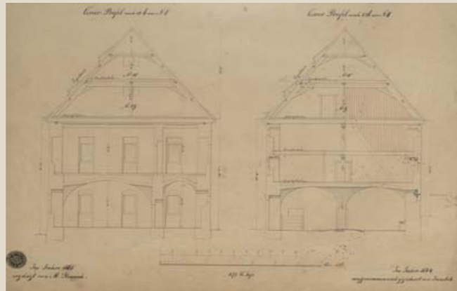
Detail řezu sýpkou na výkresové dokumentaci M. Straucha k úpravě dvora v roce 1867. (SOA v Plzni, pracoviště Klášter u Nepomuka, Vs Chotěšov, inv. č. 3416, M 557)
