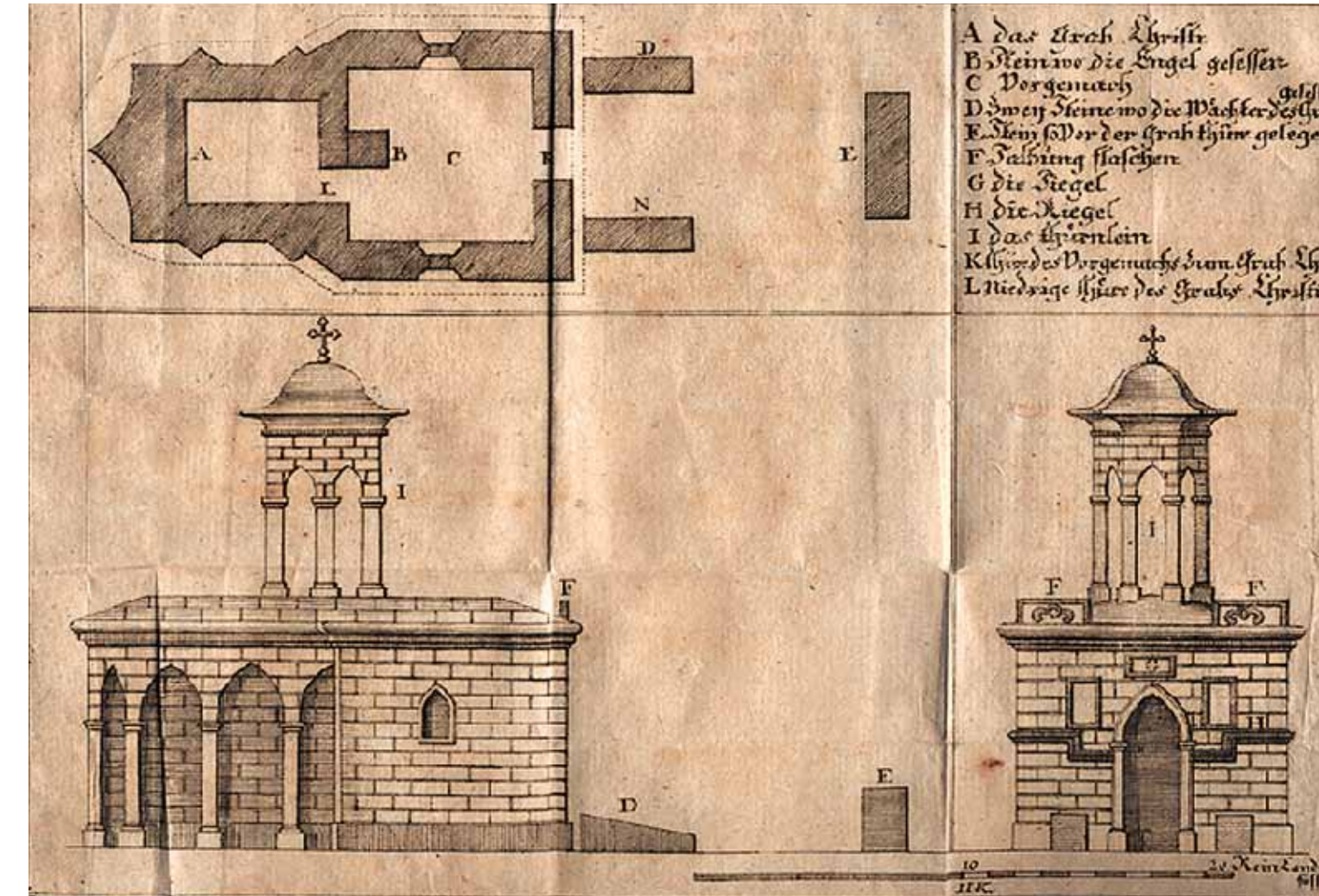
Plan der Heilig-Grab-Kapelle von 1772, der in dem Werk Gruendliche Beschreibung des in der Stadt Reichenberg Buntzlauer Creyses neu-erbauten Heiligen Grabes veröffentlicht wurde.
