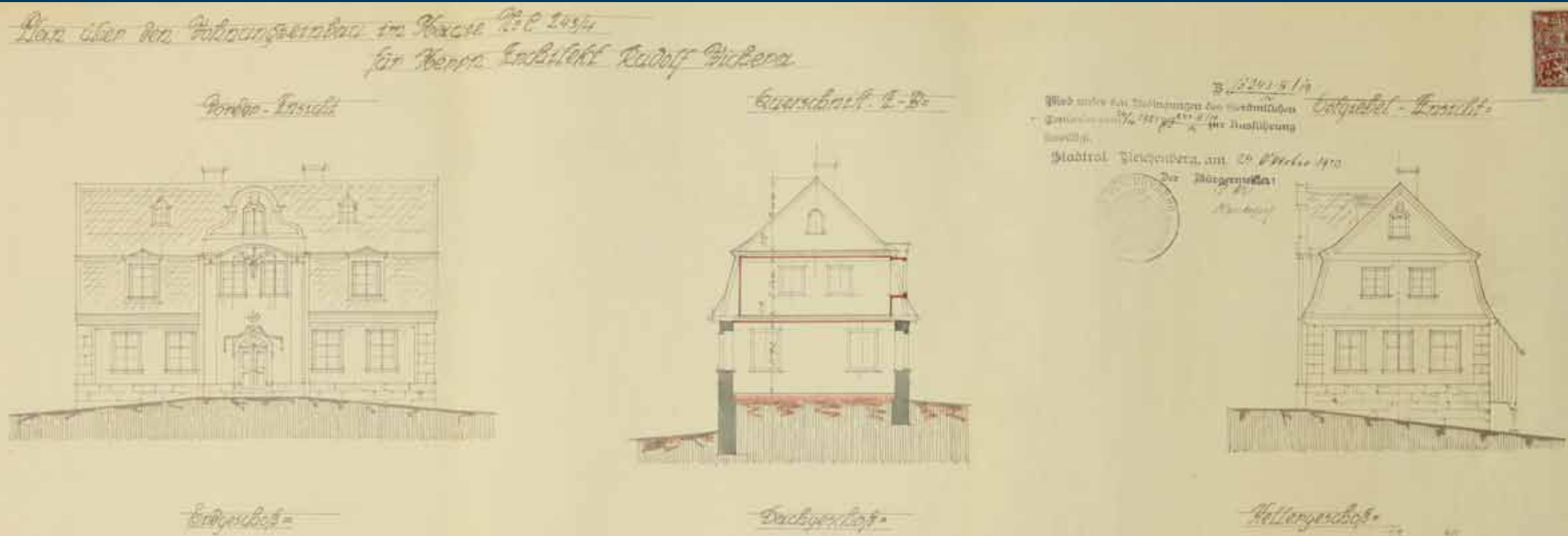
Im Liberecer Bauarchiv aufbewahrter Plan der baulichen Veränderungen des Hauses U Pelikána aus dem Jahr 1923.
